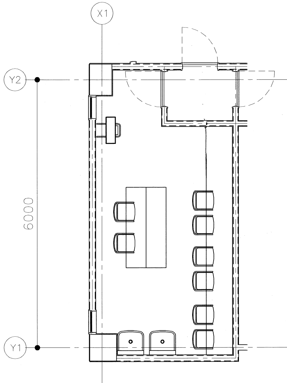
楽 屋 縮尺 1 : 50
